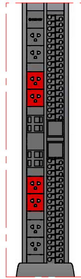
DETALLE A
